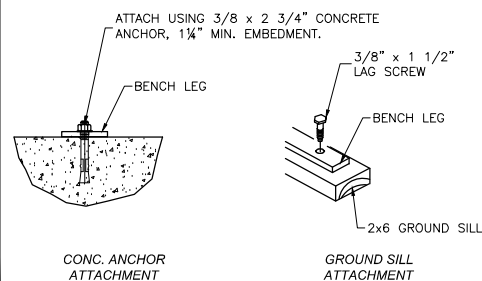
③ TYP ANCHORING DETAIL
