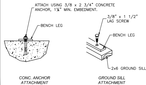
TYP ANCHORING DETAIL
